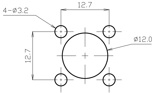
取付け穴参考寸法
