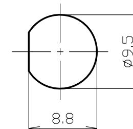
取付穴参考寸法図
