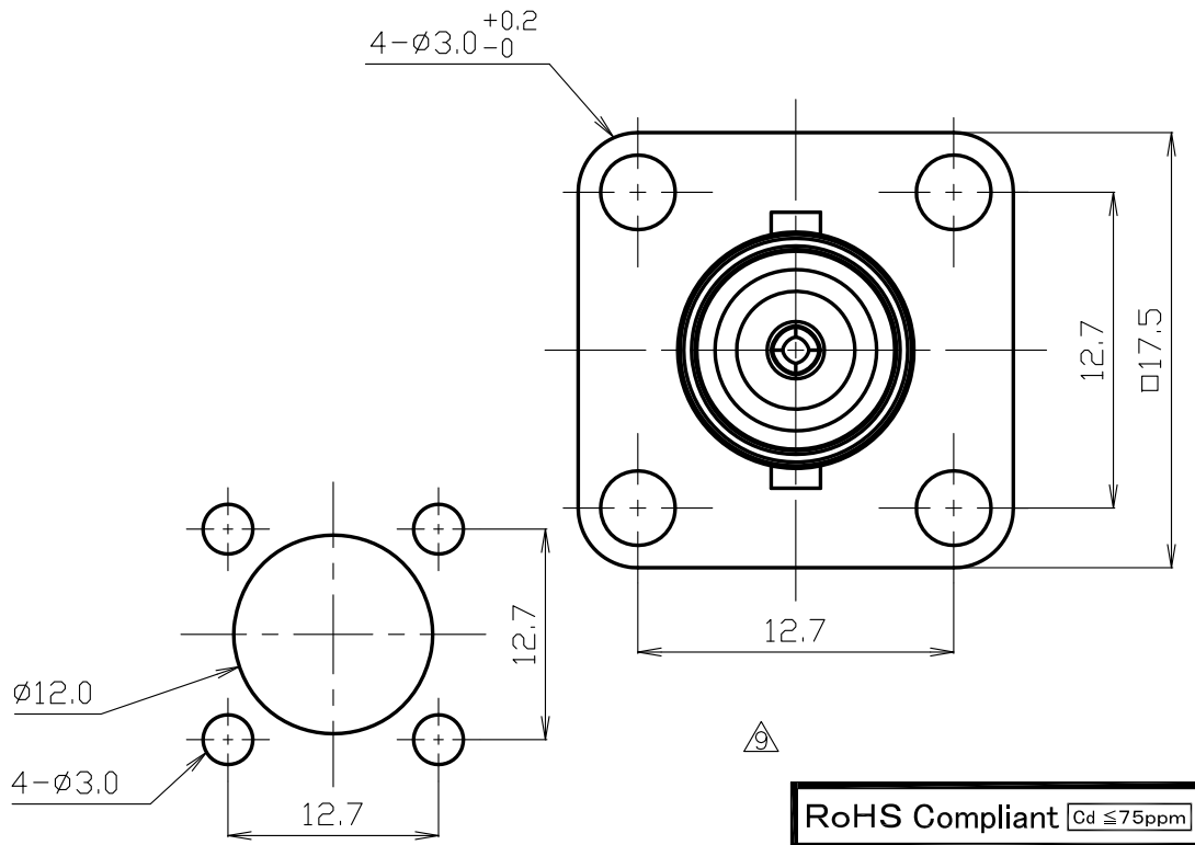
△ 取付穴参考寸法(尺度2/1)
